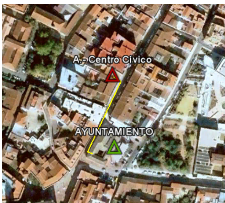
Figura 4. Despliegue de Fibra Óptica Ayuntamiento – Centro Cívico
